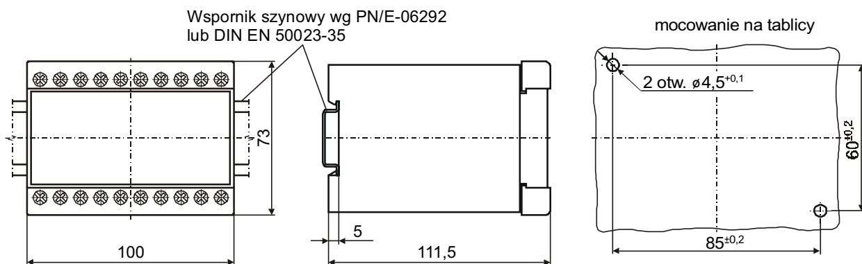
Rys. 2. Wymiary gabarytowo-montażowe przetworników mocy
